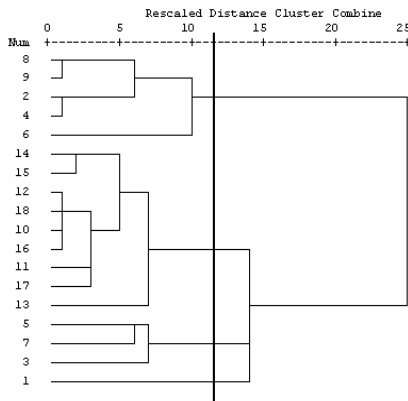
شکل ۲: دندروگرام روش دورترین همسایه‌ها
