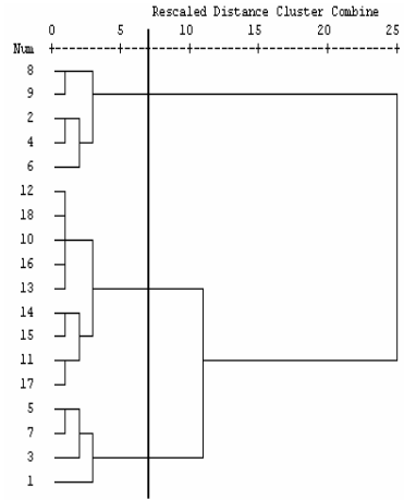
شکل ۱: دندروگرام روش حداقل واریانس وارد
