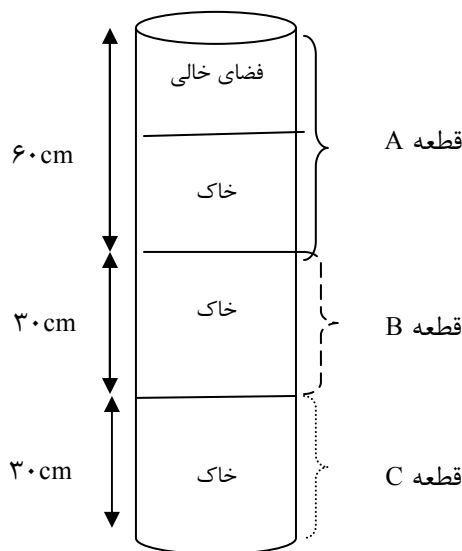
شکل ۲: نمای شماتیک لوله‌های پولیکا (PVC) در آزمایشگاه دانشکده مهندسی علوم آب
